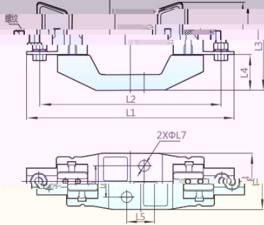
4.2.2 熔断器底座尺寸
