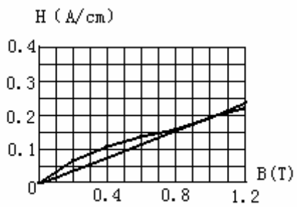
图14 D340铁心B-H曲线
