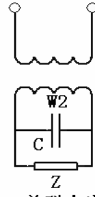
图20 并联电容补偿
